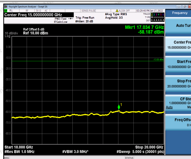
Band2-9538-1-10000~20000MHz
