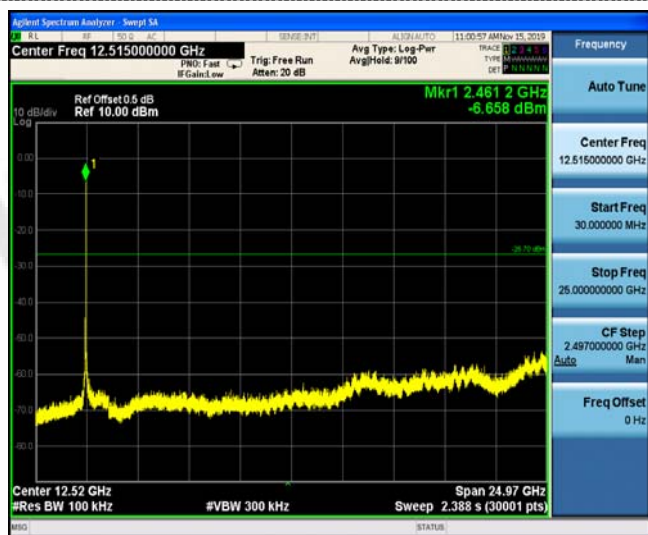
802.11n(HT20) CH11
