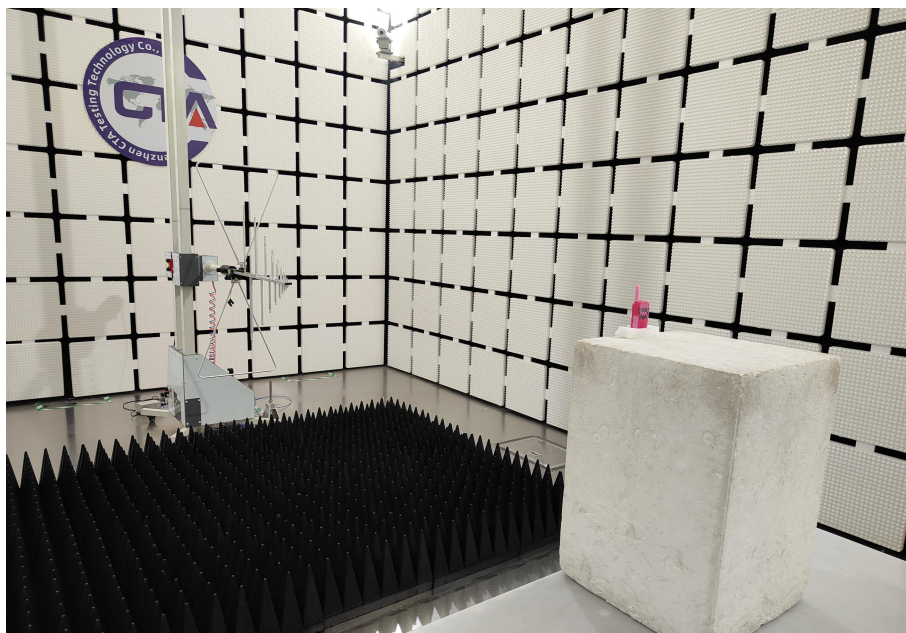
Fig. 1(Below 1GHz)
