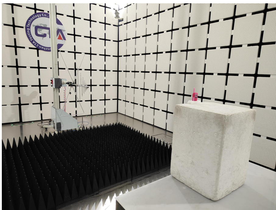
Fig. 2 (Above 1GHz)
