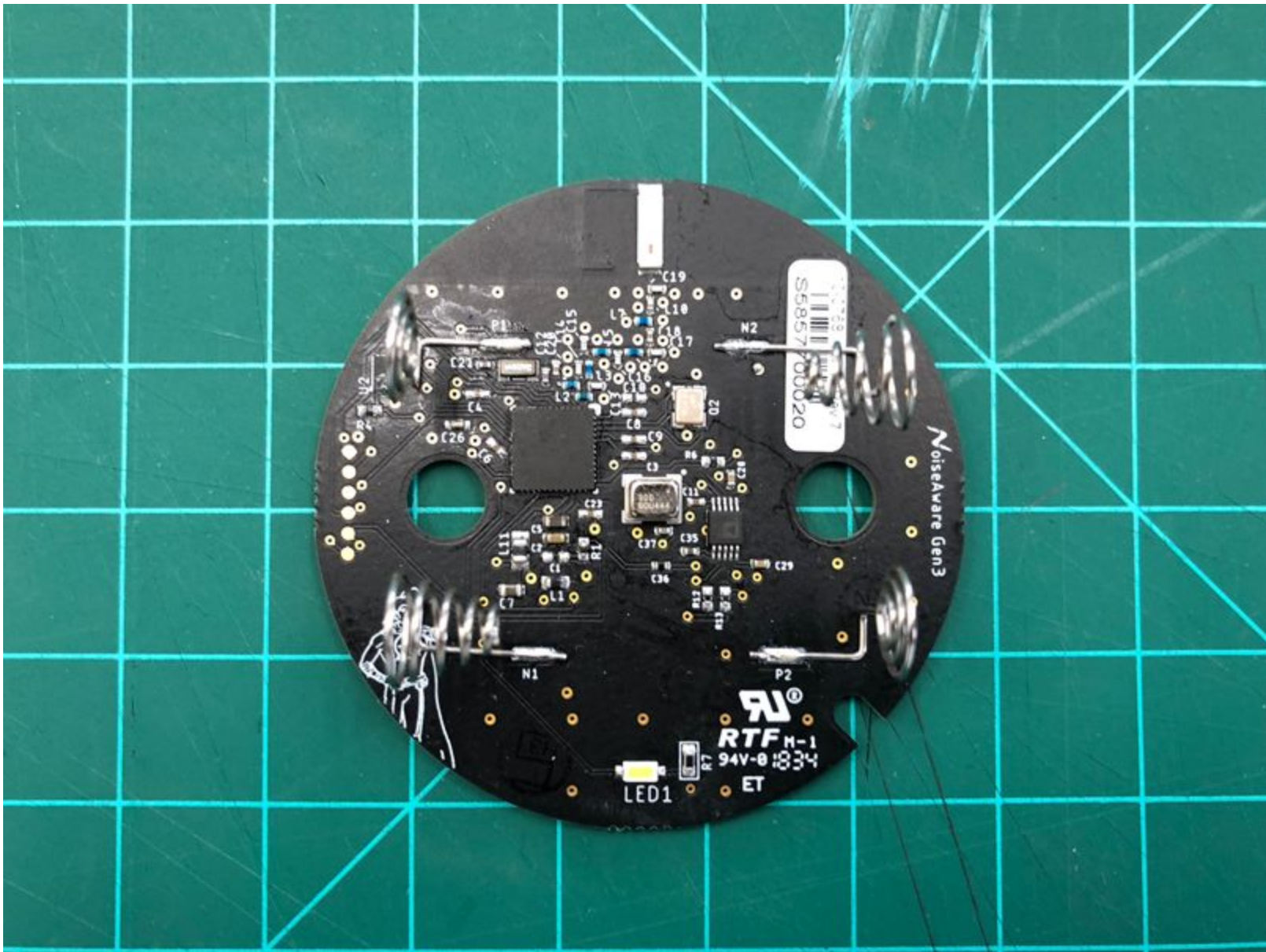
Gen3 Node - PCBA Top
