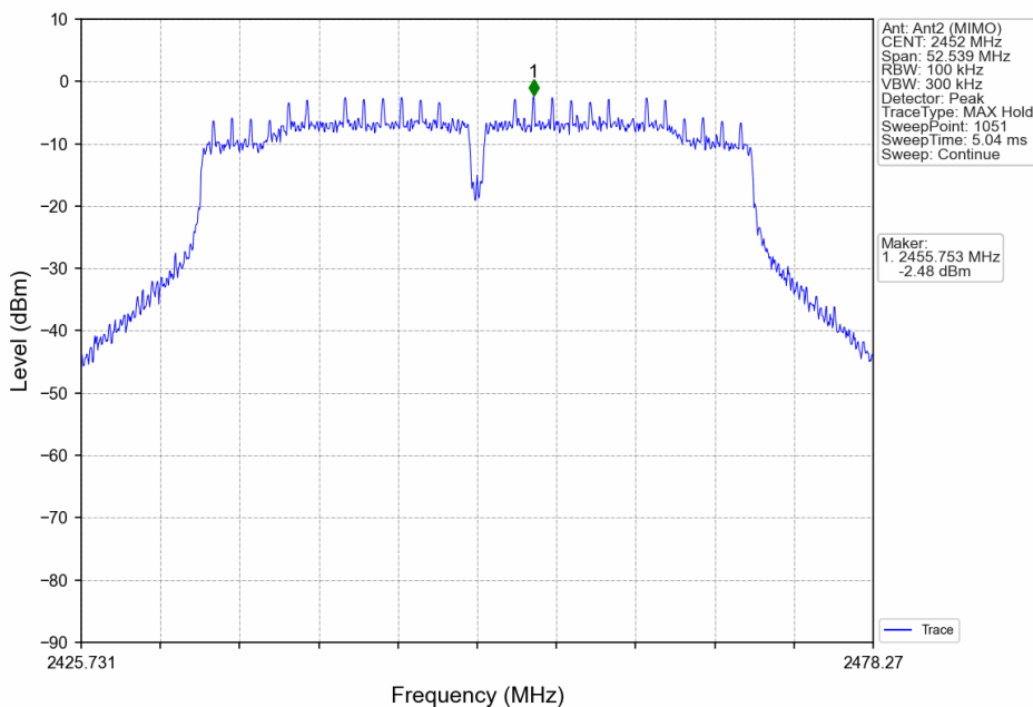
802.11n(HT40)_HCH_2452MHz_Ant2 (MIMO)_NTNV
