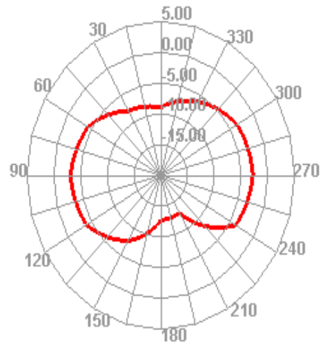
2440.000MHz E2
