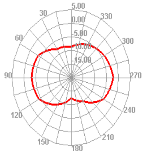
2400.000MHz E2
