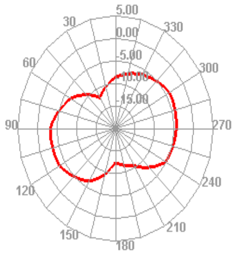
2400.000MHz E1
