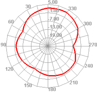
2400.000MHz H
