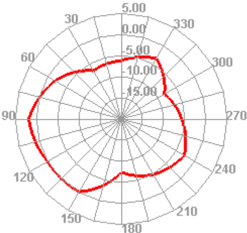
2440.000MHz E1
