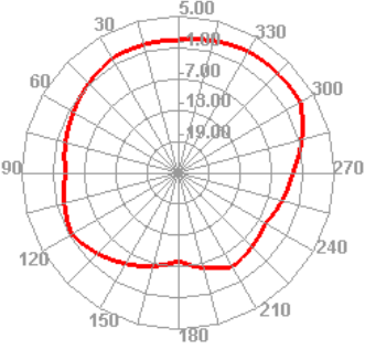
2480.000MHz H
