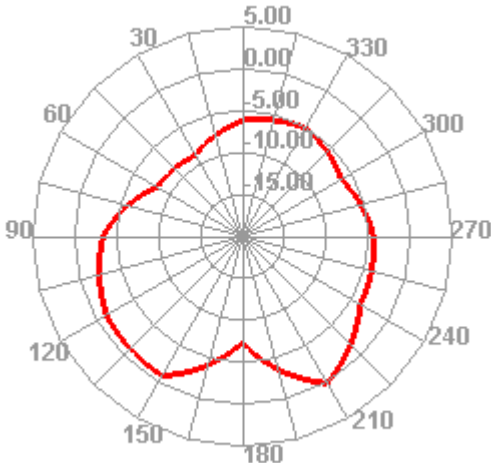
2440.000MHz E2
