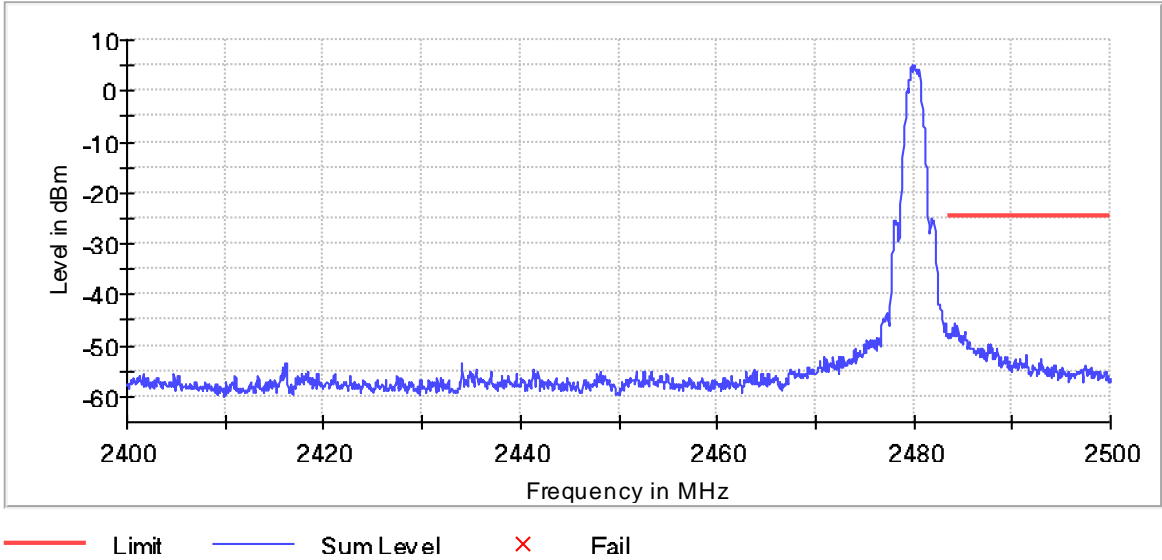
Band Edge
