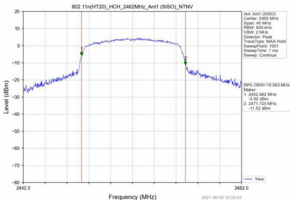
802.11n(HT20)_HCH_2462MHz_Ant1 (SISO)_NTNV
