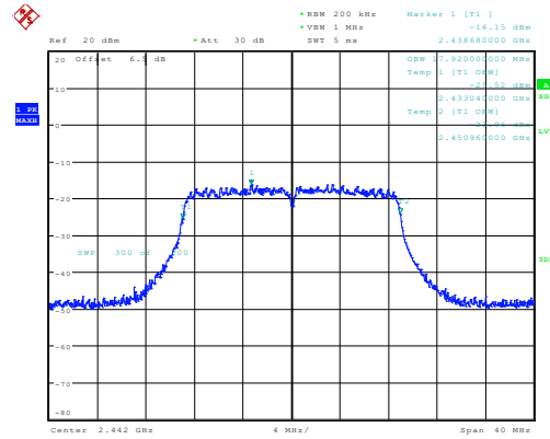
n20_2442MHz_Chain 0 17.920MHz
