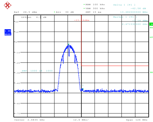
b_2472MHz_Chain 0 42.58dB
