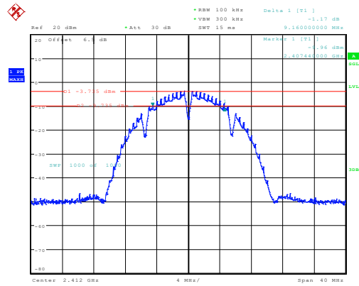
b_2412MHz_Chain 0 9.160MHz
