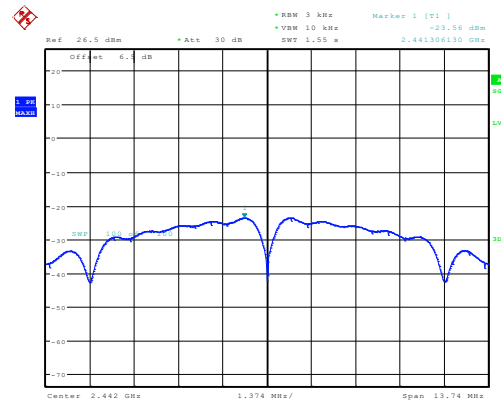
b_2442MHz_Chain 0 -23.56dBm/3kHz
