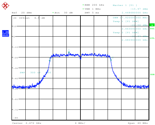
n20_2472MHz_Chain 0 17.920MHz
