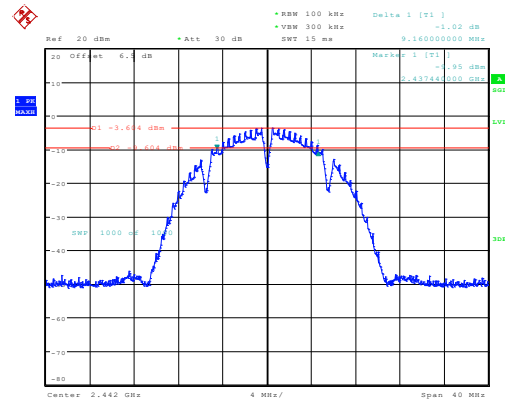
b_2442MHz_Chain 0 9.160MHz
