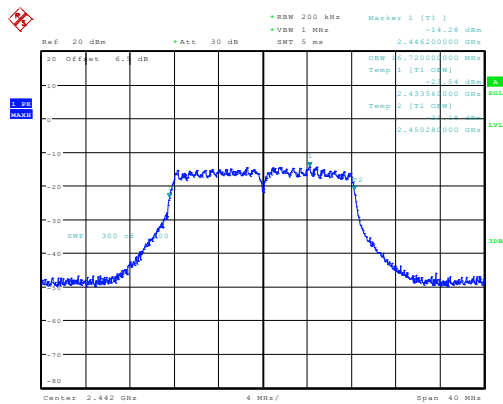
g_2442MHz_Chain 0 16.720MHz
