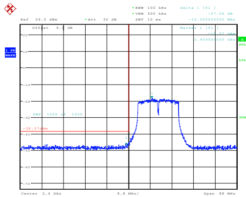
g_2412MHz_Chain 0 27.06dB
