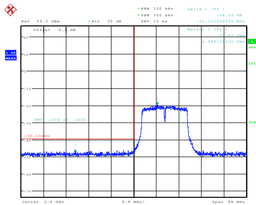
n20_2412MHz_Chain 0 26.39dB
