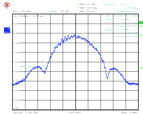
High 1.998MHz
