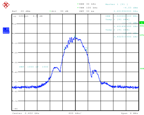
Low 1.020MHz
