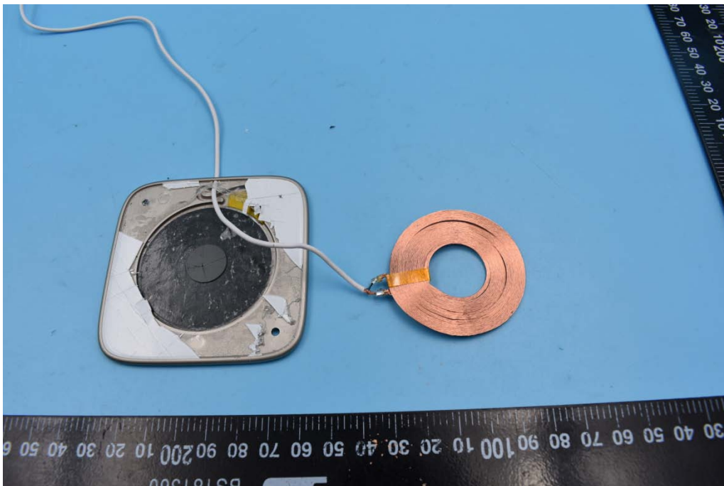
Model No:LXWCD01B
