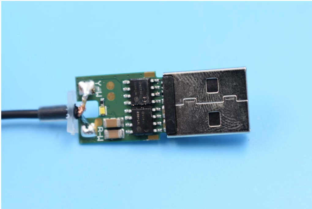
Model No:LXWCD02C
