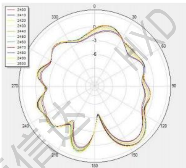
V Phi=0
