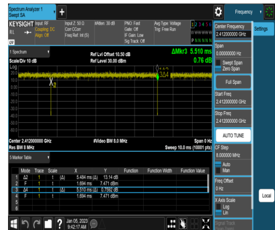
802.11n HT40
