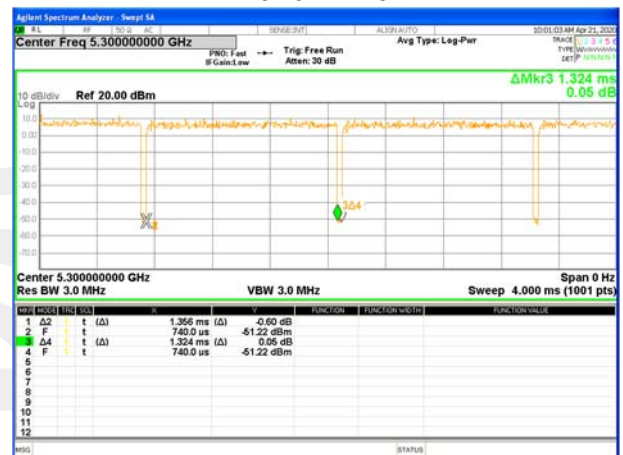
Band 2-ac20
