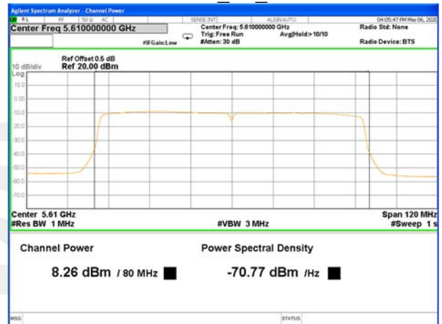
5610MHz_AV_Ant A
