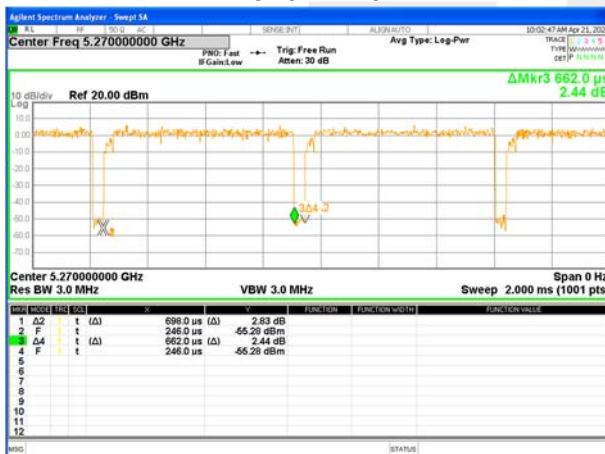
Band 2-ac40
