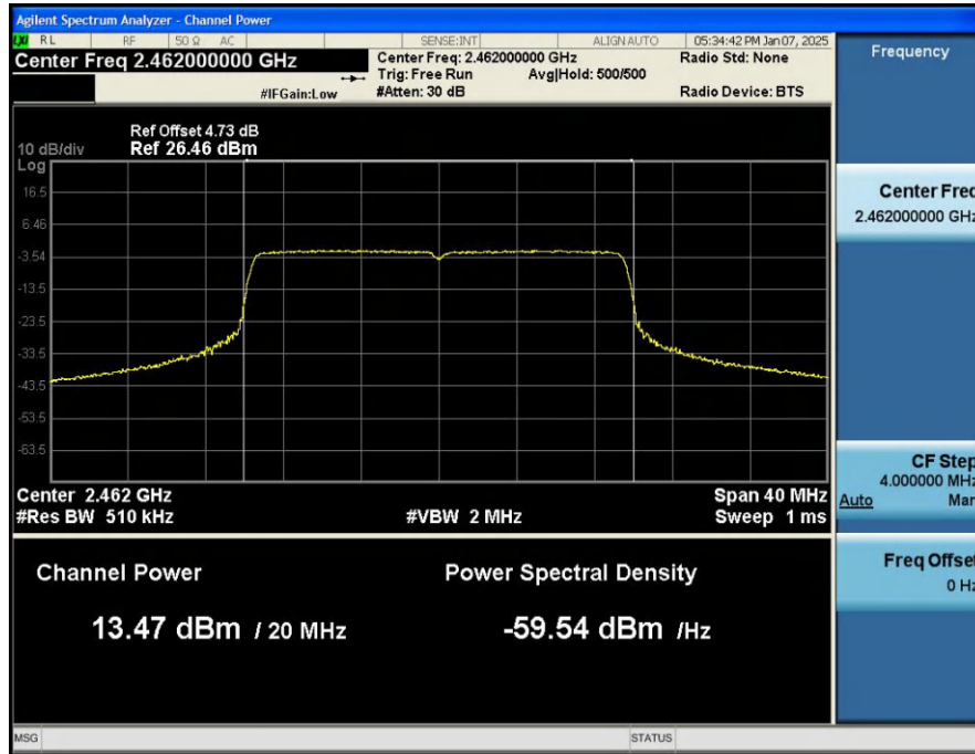
MAX__Output_Power_NVNT_ANT1_802_11ax(HE20)_2462
