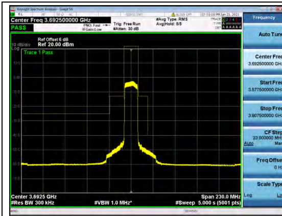
B48-15M-MASK-H-Q64
