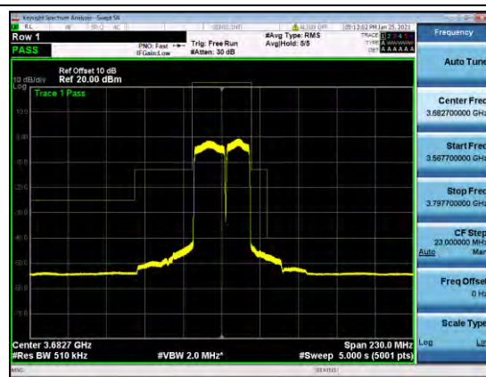
B48-20-15-MASK-H-Q64
