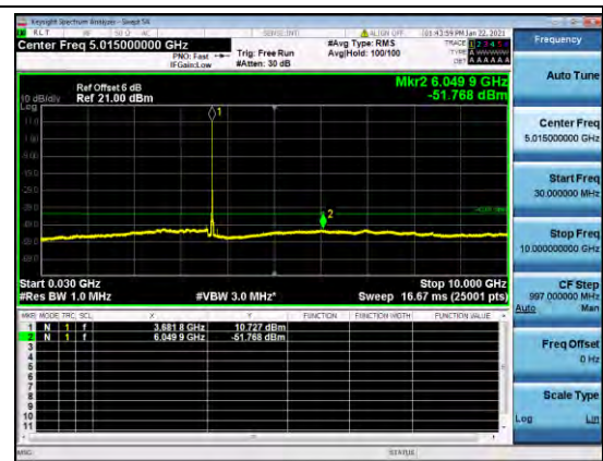
B48-20M-CSE-H-Q64-3
