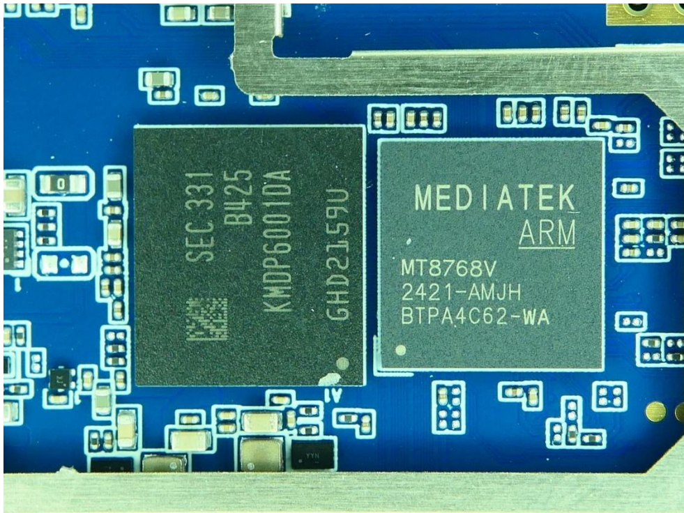
(20) EUT Photo
