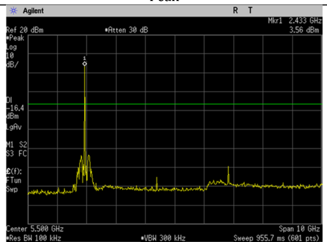
Mid Ch_2440MHz_2MBit_-20dBc_30MHz-10GHz
