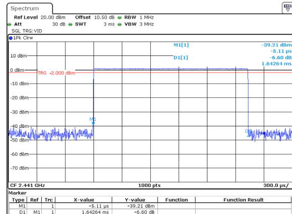
DH3_Hopping 1.643ms
