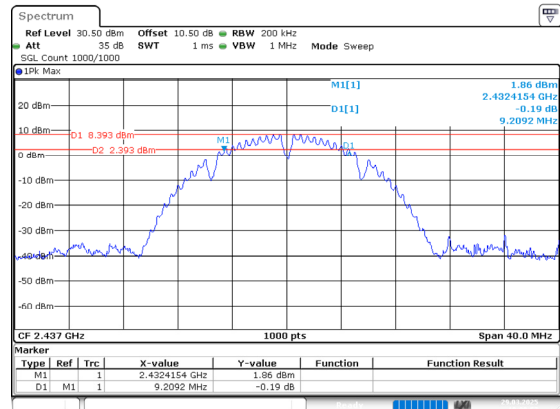
802.11b_2437MHz_Chain 0
