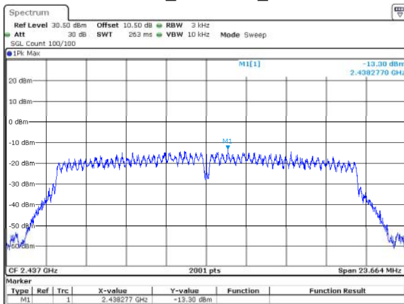
802.11n20_2437MHz_Chain 1
