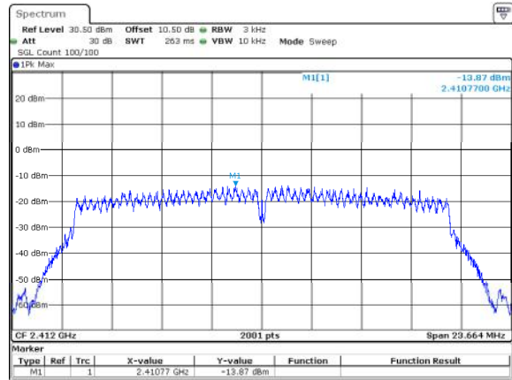
802.11n20_2412MHz_Chain 1
