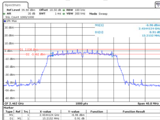
802.11n20_2462MHz_Chain 0
