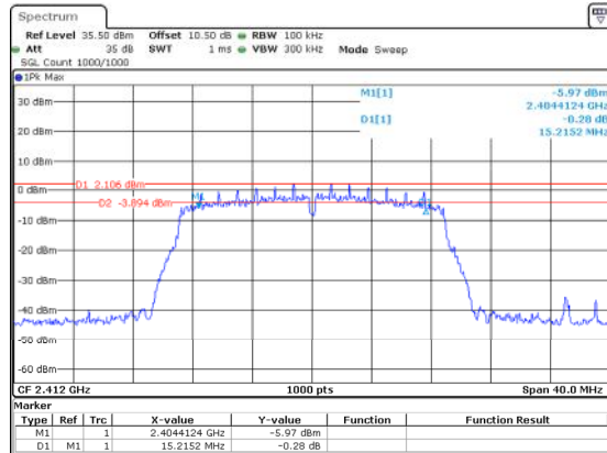
802.11n20_2412MHz_Chain 0
