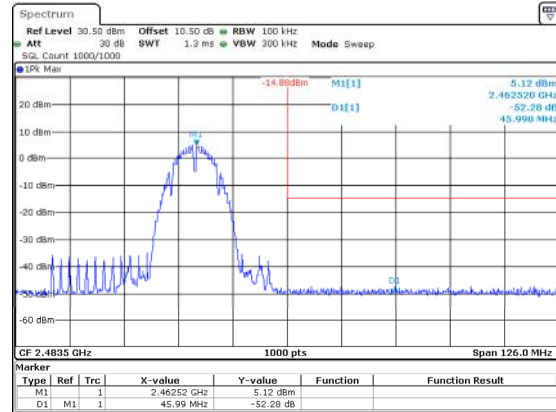
802.11b_2462MHz_Chain 0
