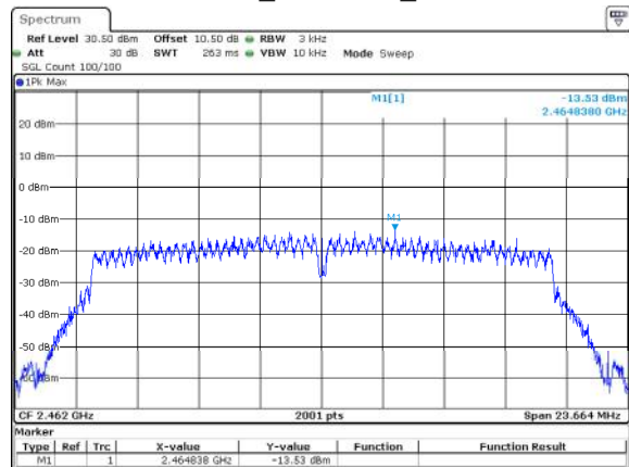
802.11n20_2462MHz_Chain 1
