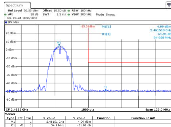
802.11b_2462MHz_Chain 1
