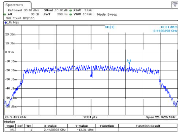
802.11n20_2437MHz_Chain 0
