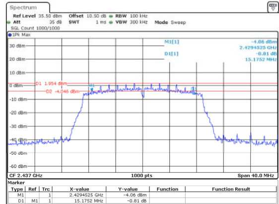
802.11n20_2437MHz_Chain 0
