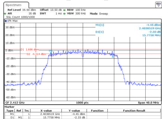
802.11n20_2412MHz_Chain 1
