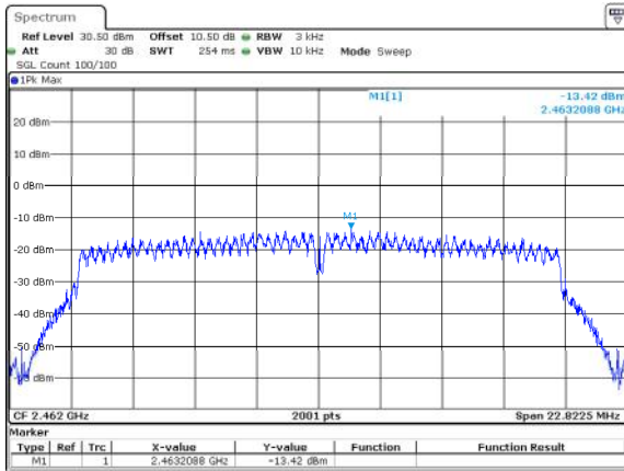
802.11n20_2462MHz_Chain 0
