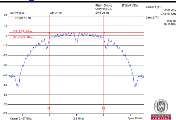
802.11b_CH6
