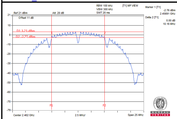
802.11b_CH11
