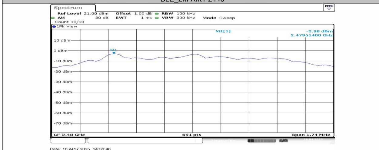
BLE_2M-Ant1-2480
