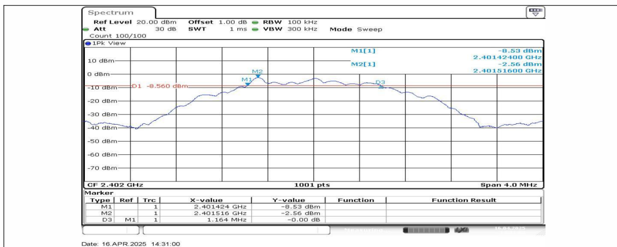
BLE_2M-Ant1-2402
