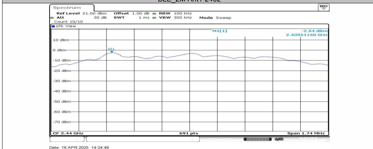
BLE_2M-Ant1-2440
