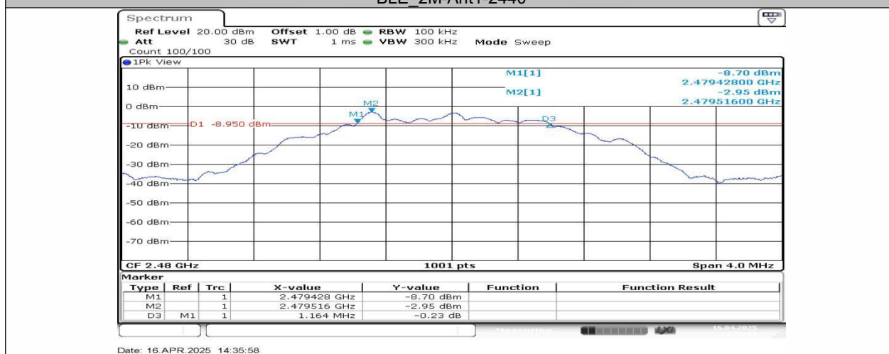
BLE_2M-Ant1-2480
