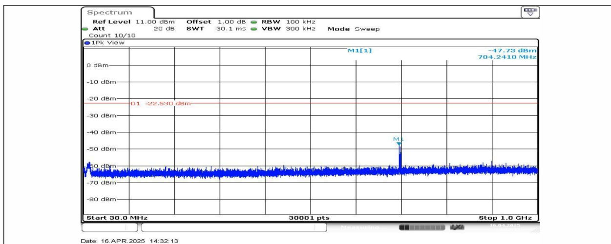
BLE_2M-Ant1-2402-30~1000
