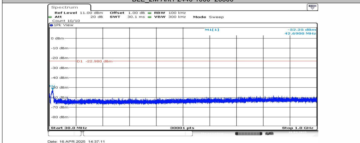
BLE 2M-Ant1-2480-30~1000
