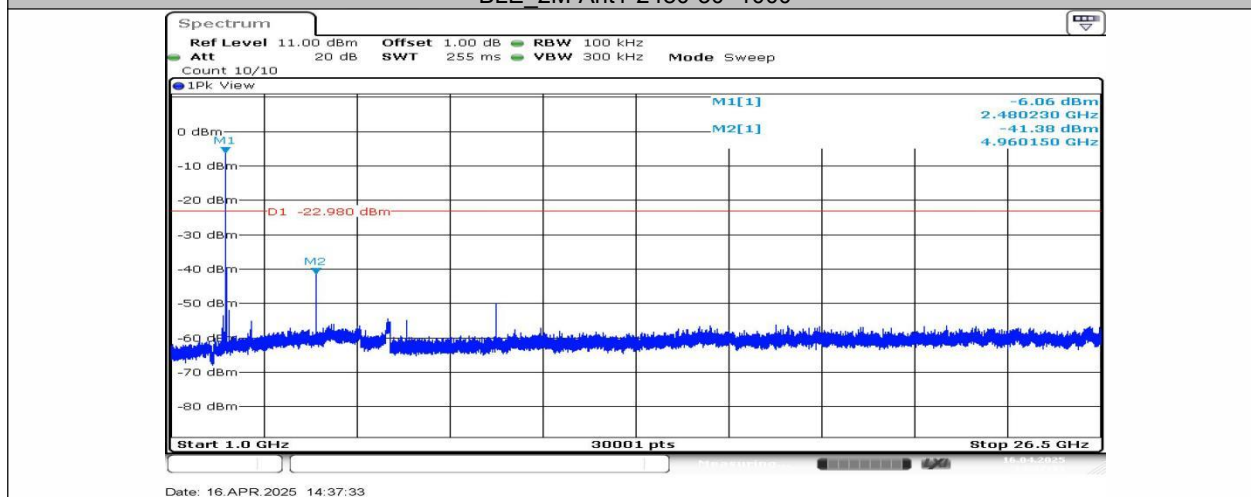
BLE 2M-Ant1-2480-1000~26500
