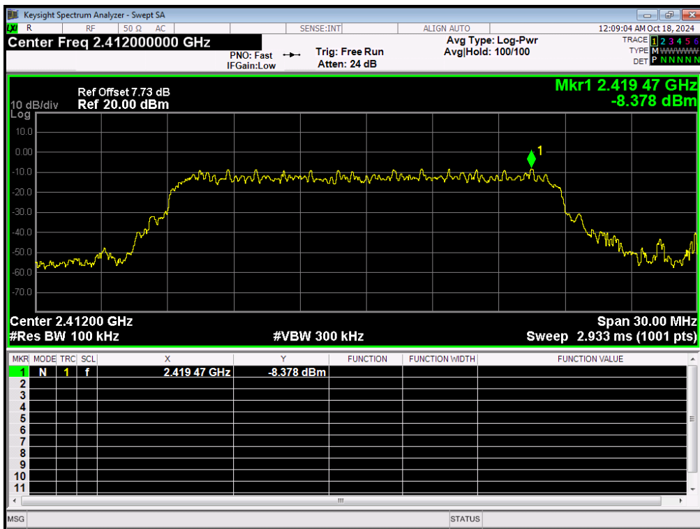
Band Edge NVNT 802.11g 6Mbps 2412MHz Ant1 Ref
