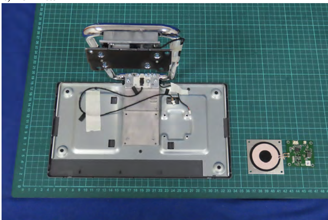
(16) EUT Photo
