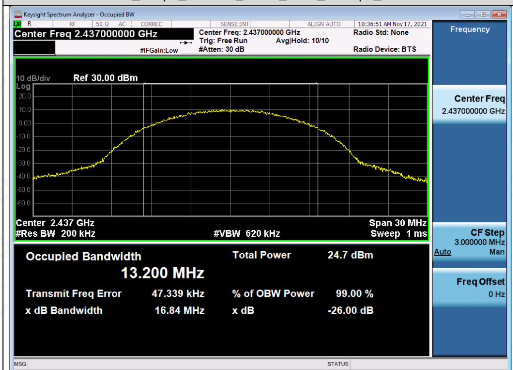
Test_Graph_802.11b_ANT1_2437_11Mbps_OBW
