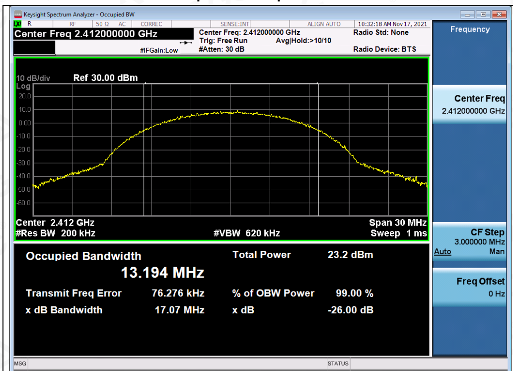
Test_Graph_802.11b_ANT1_2412_11Mbps_OBW
