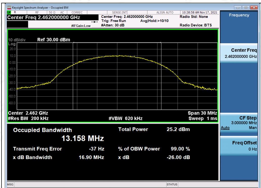
Test_Graph_802.11b_ANT1_2462_11Mbps_OBW
