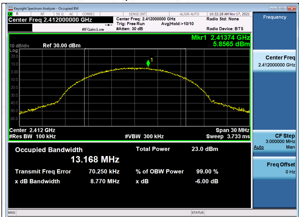
Test_Graph_802.11b_ANT1_2412_11Mbps_DTSBW
