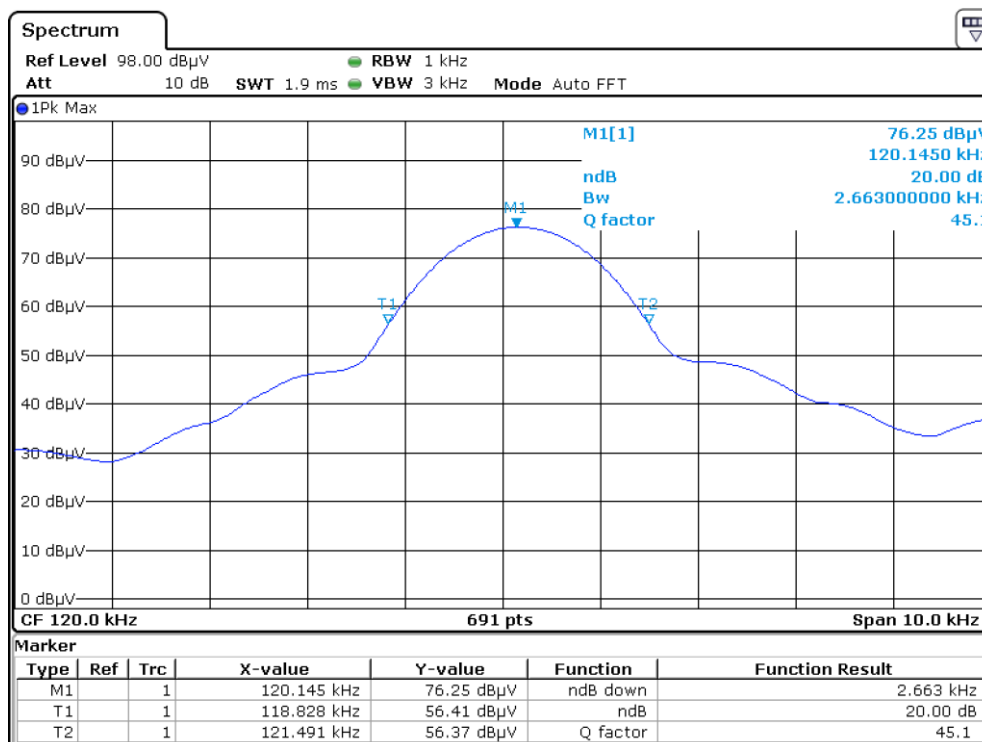
Output B
