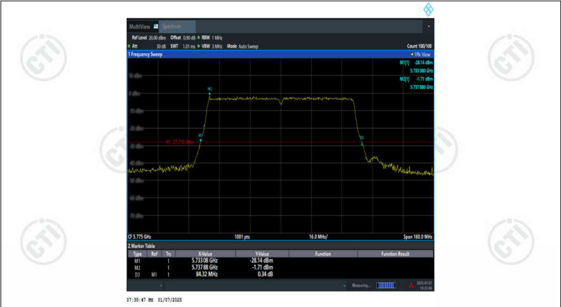
11AC80SISO-Ant1-5775
