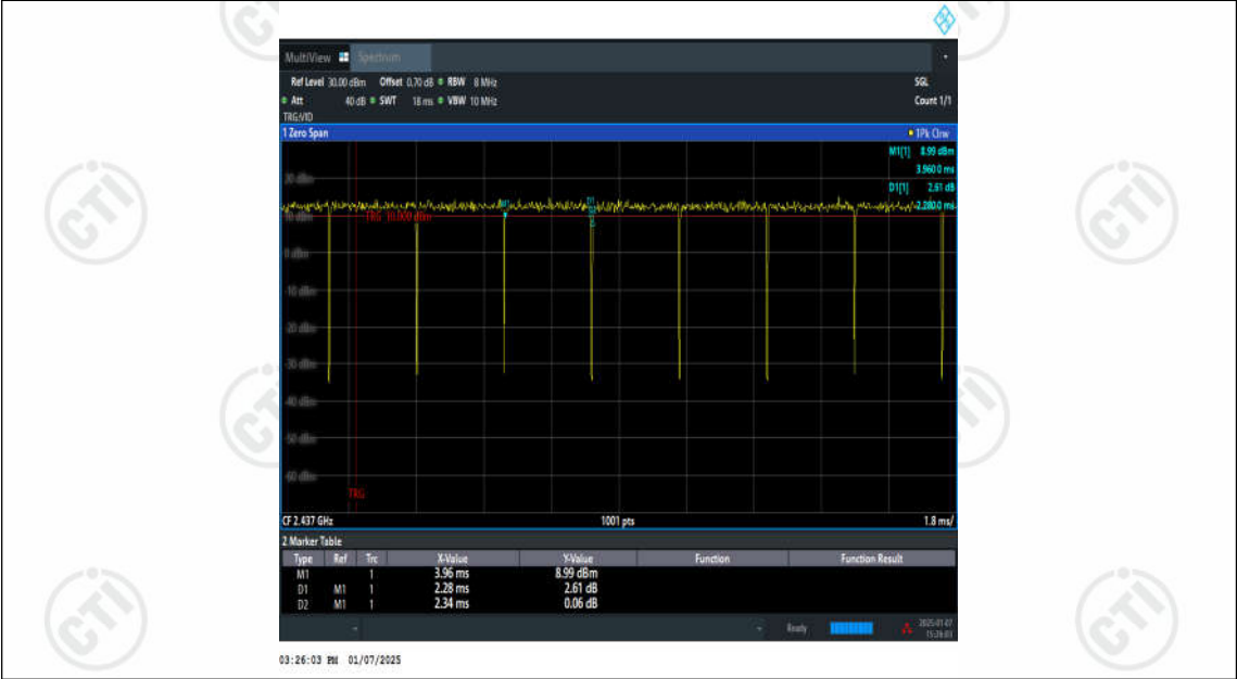
NTNV-11AX20MIMO-Ant2-2437
