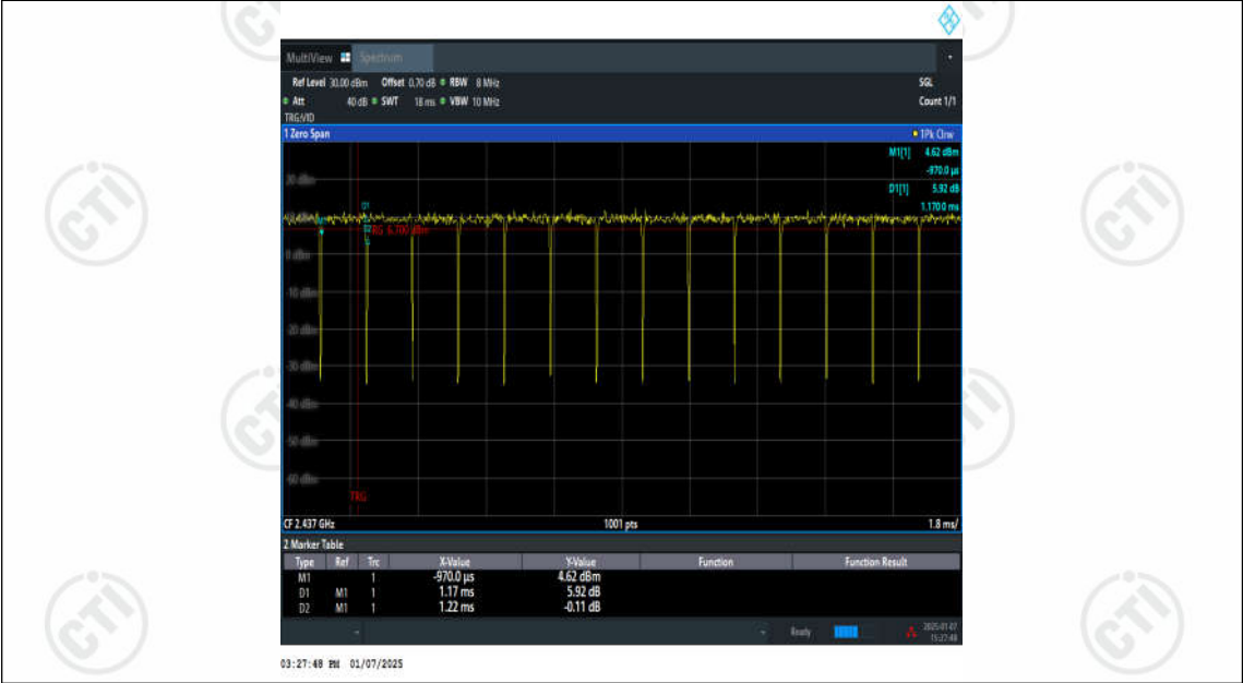
NTNV-11AX40MIMO-Ant2-2437
