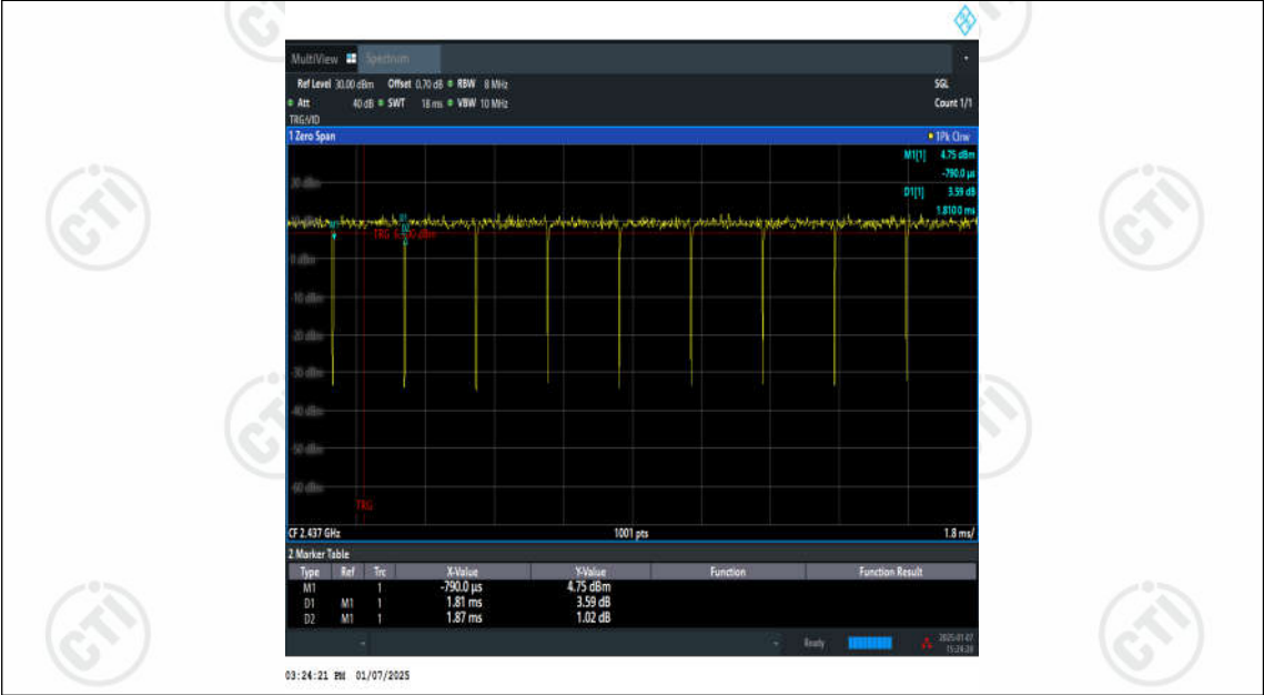
NTNV-11N40MIMO-Ant2-2437
