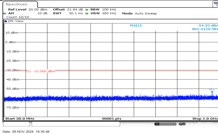
11G_Ant1_2462_30-1000
