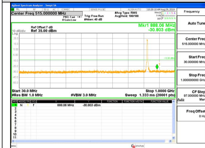
WCDMA850-LCH
