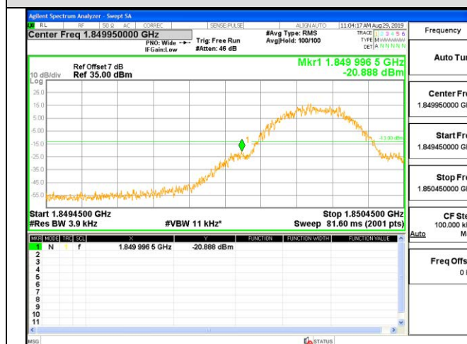
GSM 1900-LCH-GPRS
