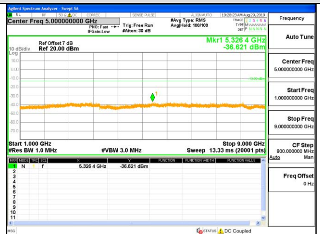
WCDMA850-LCH
