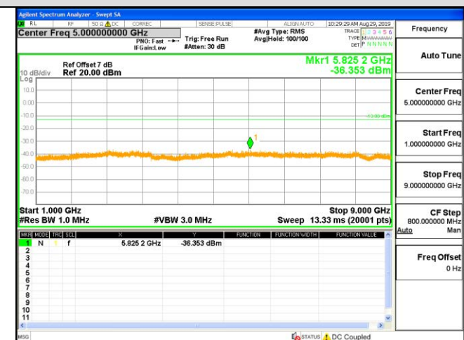
WCDMA850-HCH
