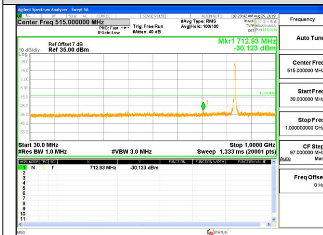
WCDMA850-MCH
