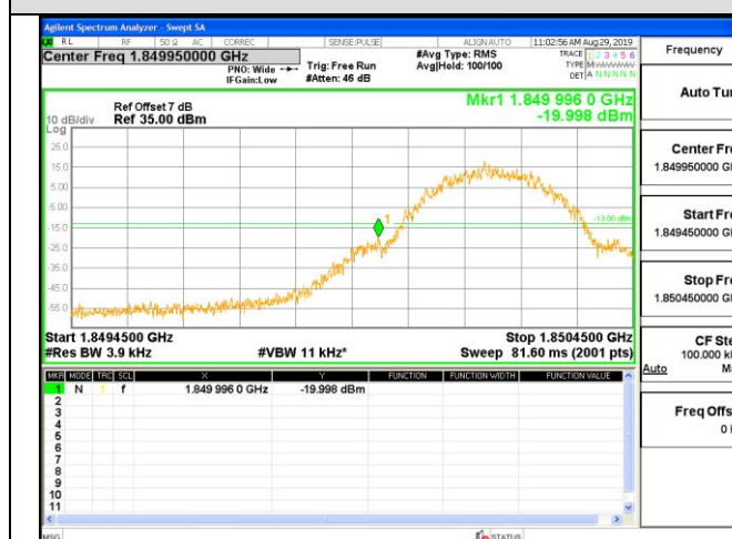
GSM 1900-LCH-GSM
