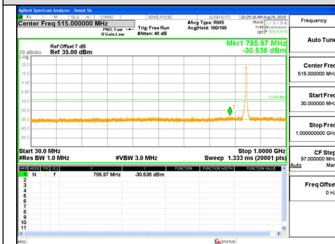
WCDMA850-HCH
