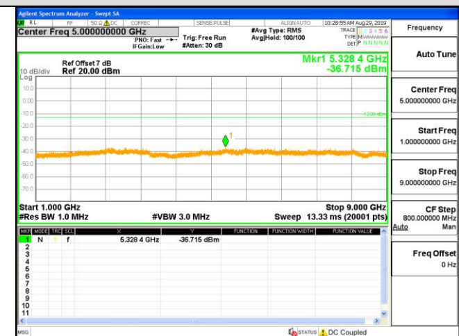
WCDMA850-MCH
