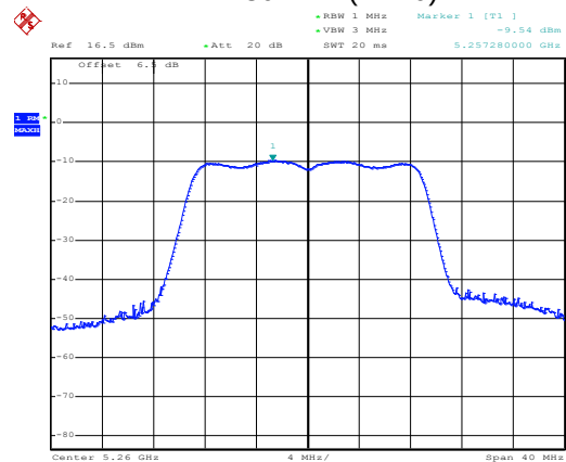
802.11n(HT20)
