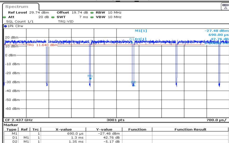
11N20SISO_Ant1_2437
