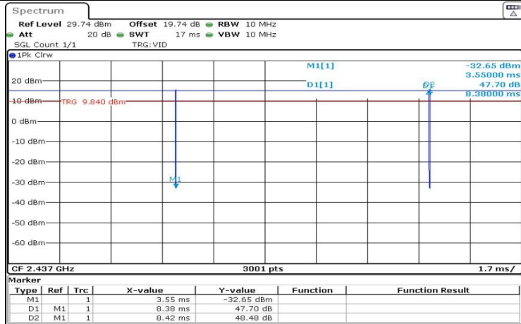
11B_Ant1_2437
