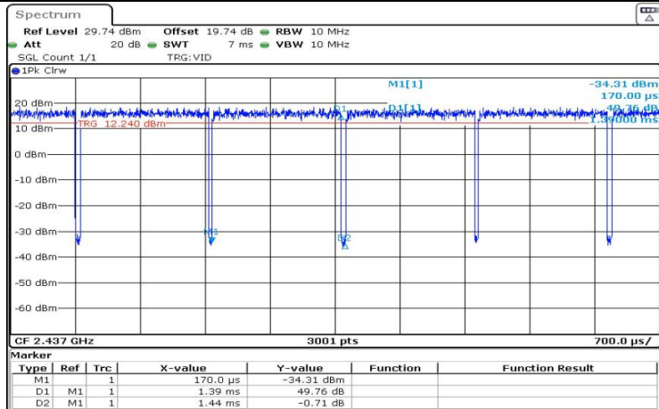
11G_Ant1_2437
