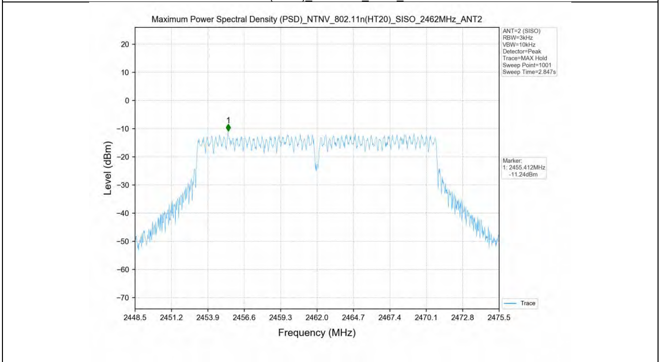
802.11n(HT20)_2462MHz_SISO_ANT2
