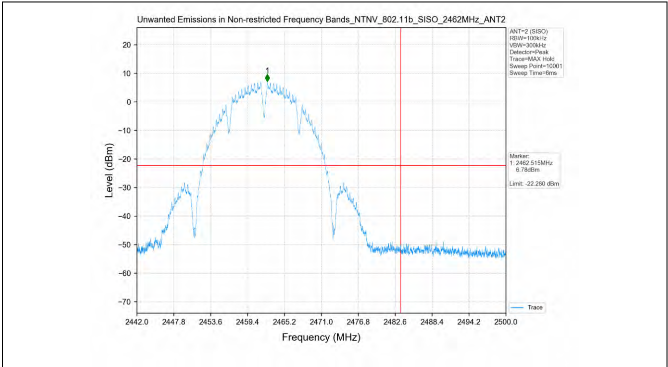
802.11b_2462MHz_SISO_ANT2
