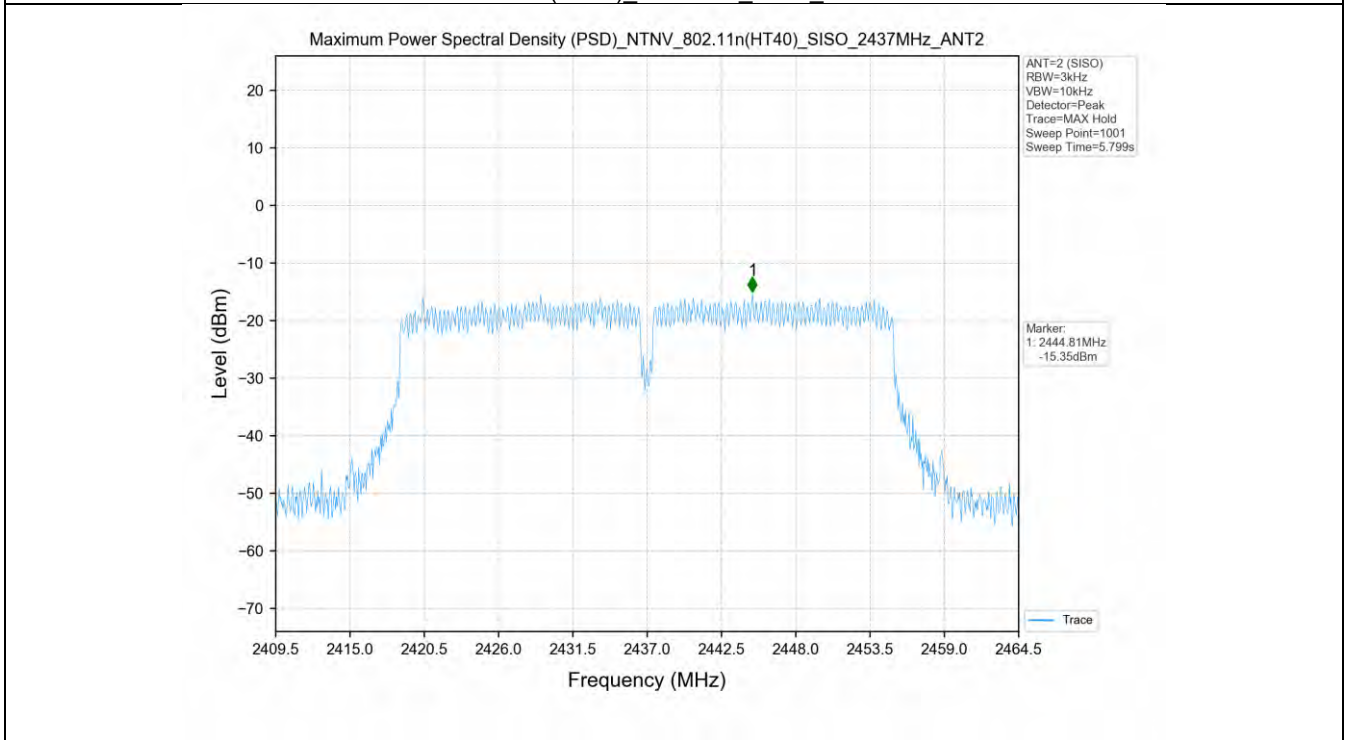
802.11n(HT40)_2437MHz_SISO_ANT2
