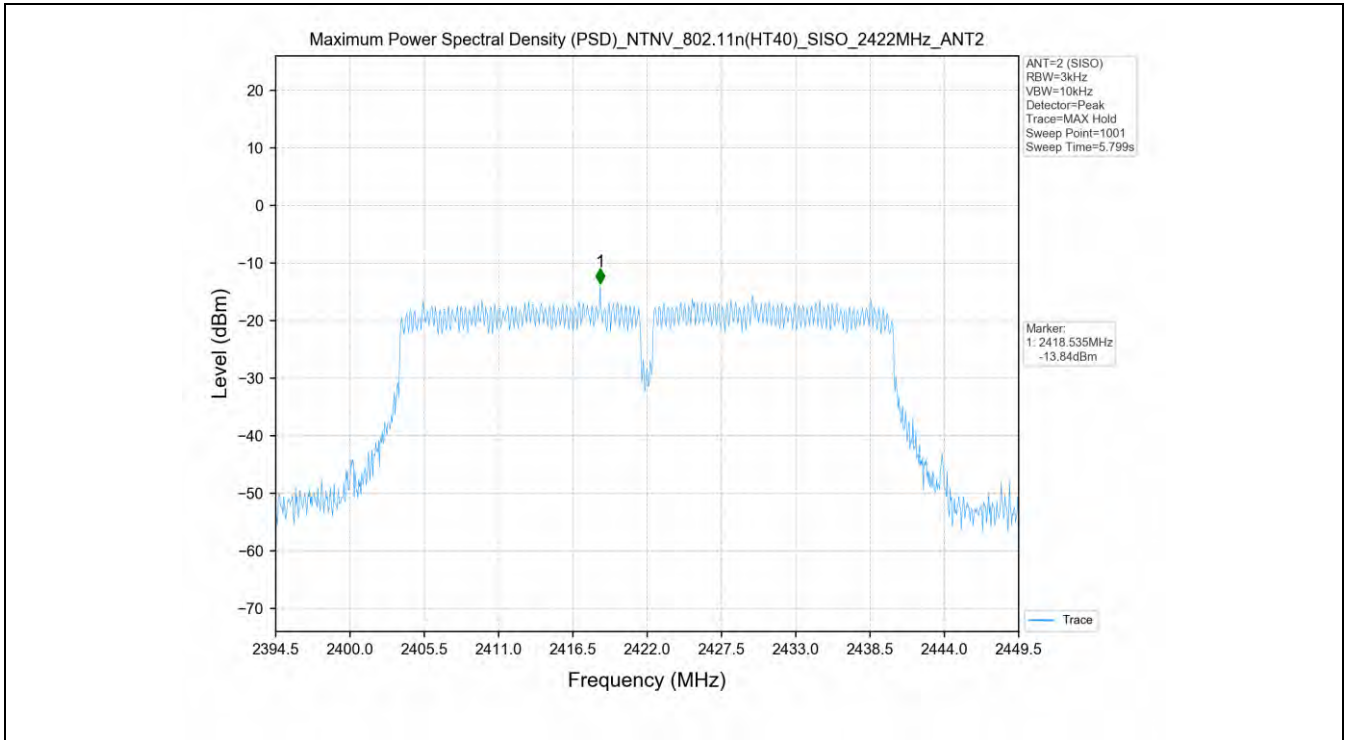
802.11n(HT40)_2422MHz_SISO_ANT2
