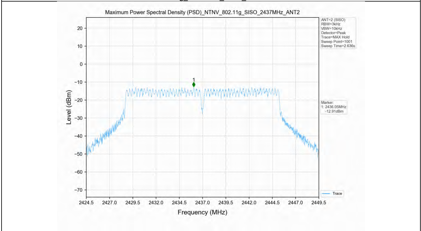
802.11g_2437MHz_SISO_ANT2
