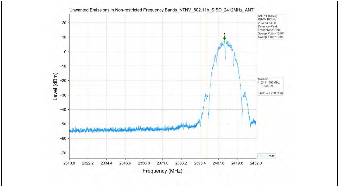
802.11b_2412MHz_SISO_ANT1
