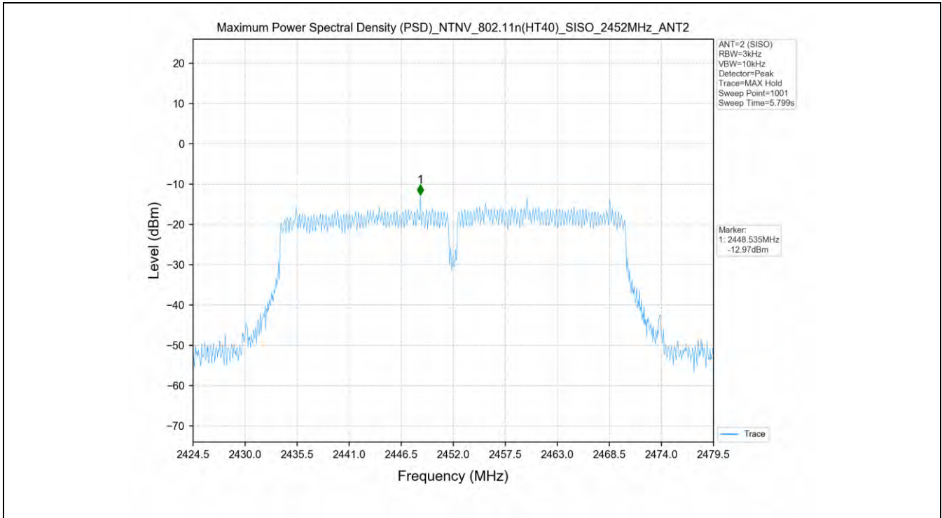
802.11n(HT40)_2452MHz_SISO_ANT2
