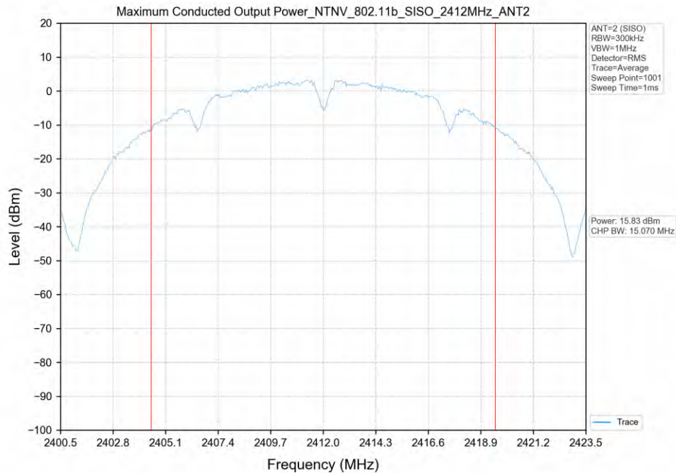
802.11b_2412MHz_SISO_ANT2
