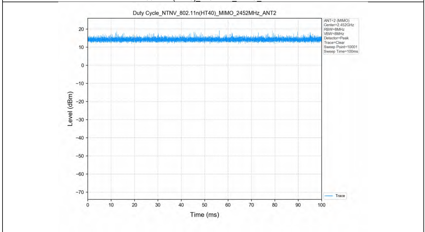
802.11n(HT40)_2452MHz_MIMO_ANT2
