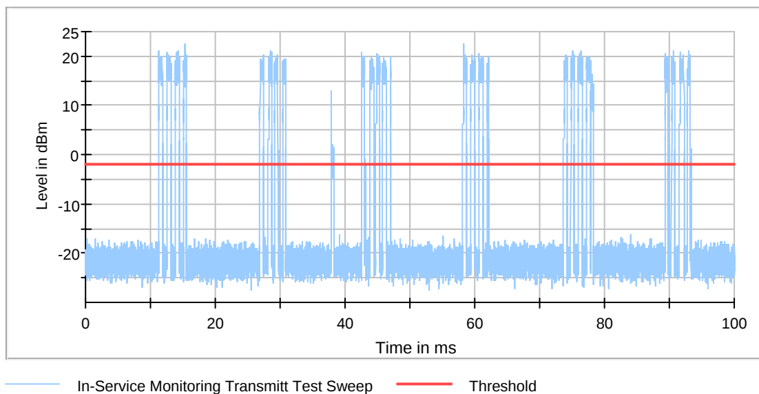
802.11ac VHT80 5610MHz
