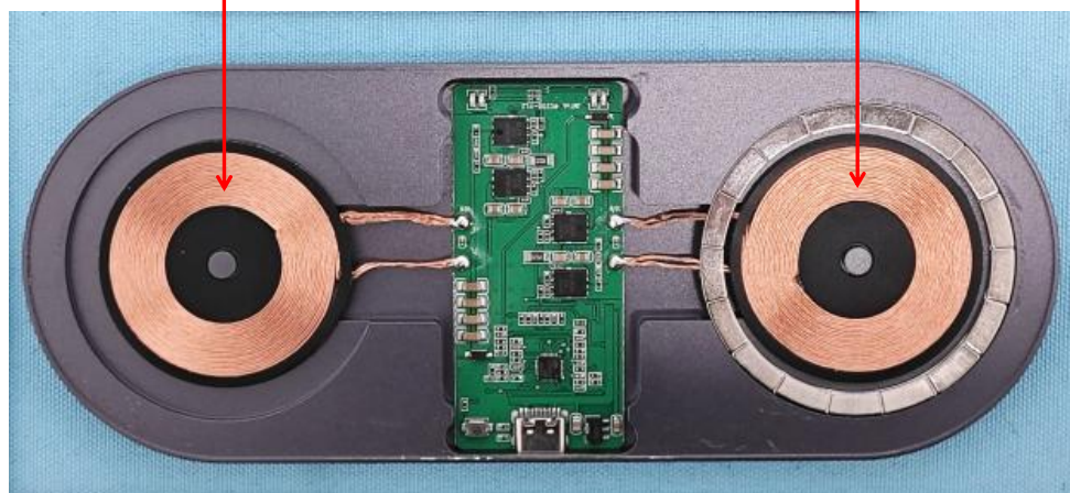
WPT-10W ANT
