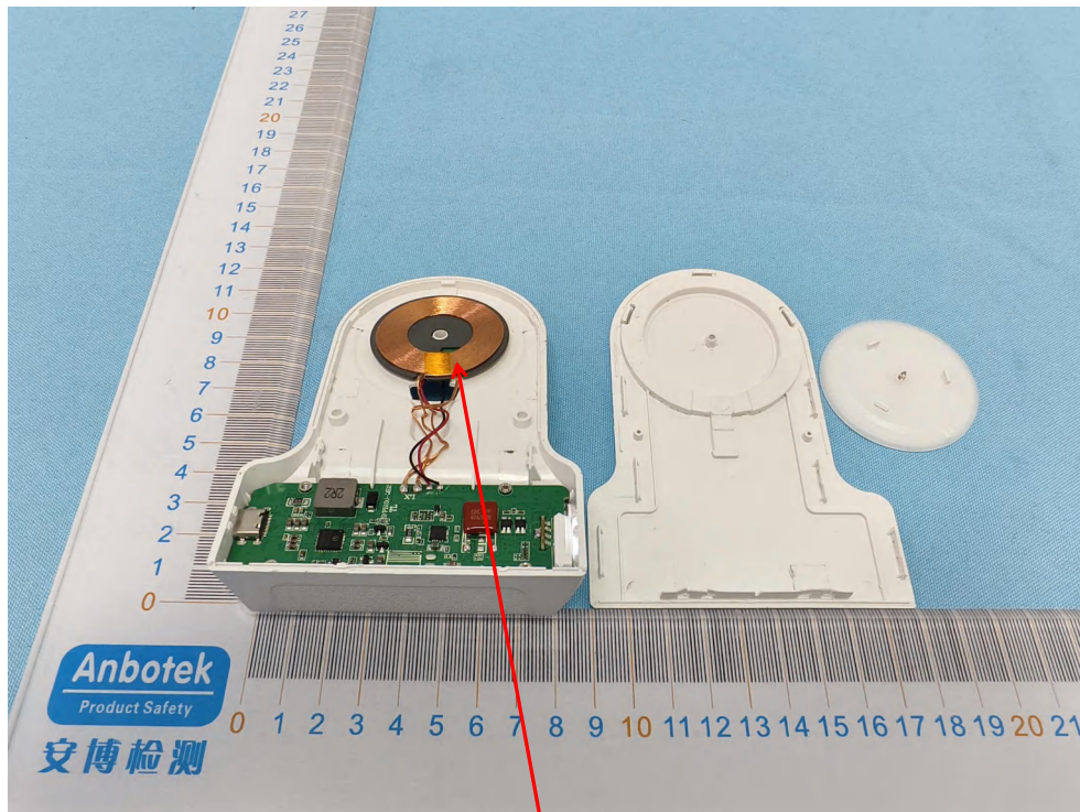
WPT-ANT
