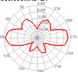
2500.000MHz E1
