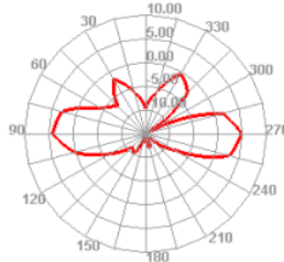
2400.000MHz E2
