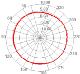
2400.000MHz H
