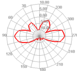
2400.000MHz E1
