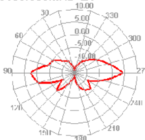
5150.000MHz E1
