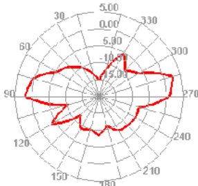
5850.000MHz E1
