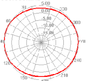
5500.000MHz H
