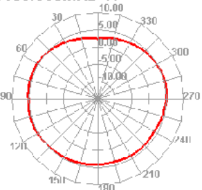
5150.000MHz H
