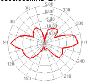
5500.000MHz E1
