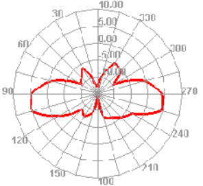
2500.000MHz E2
