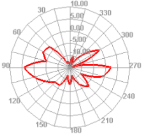
5500.000MHz E1
