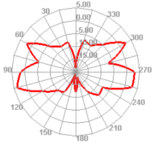
5150.000MHz E2
