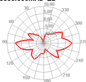
5850.000MHz E2
