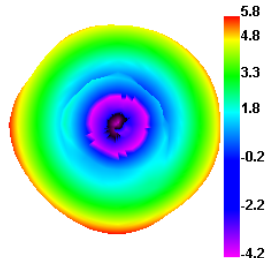
5850.000MHz
