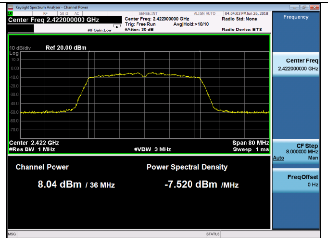
802.11n40 - PK Output power - Low CH 2422
