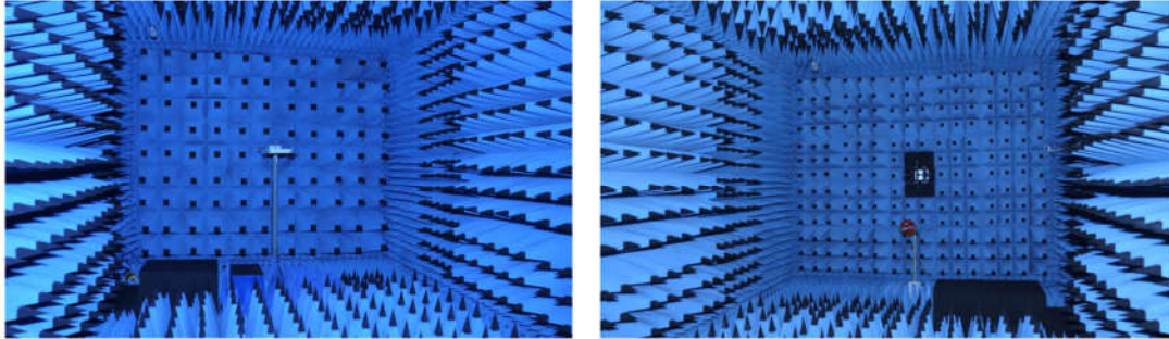
Anechoic chamber 700MHz – 6000MHz
