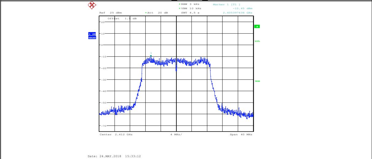
11N20 ANT2 2412
