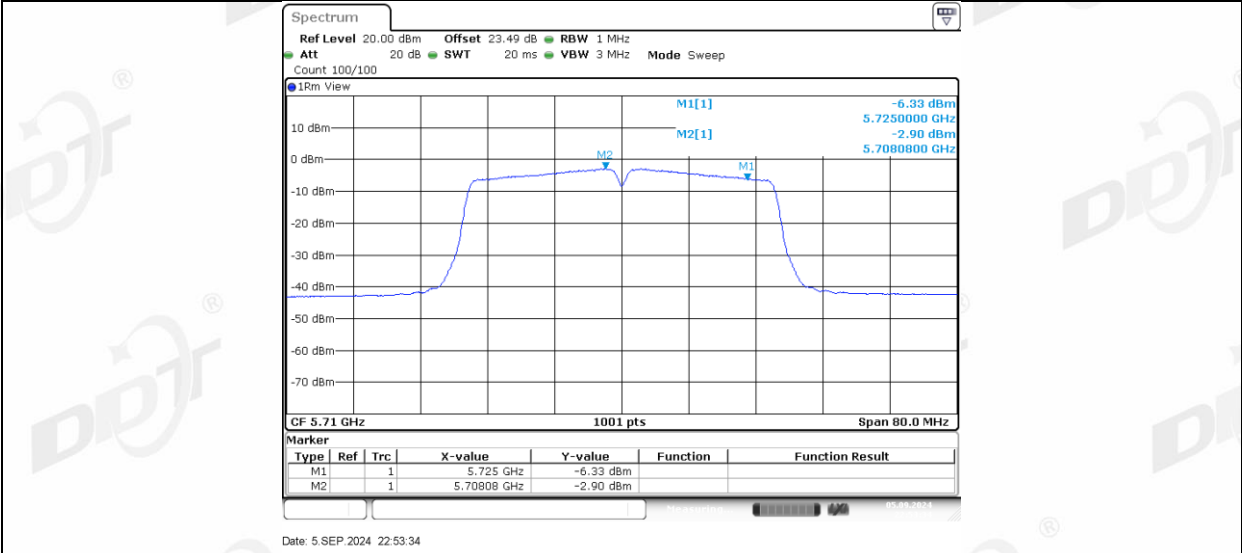
11AC40MIMO_Ant1_5710_UNII-3
