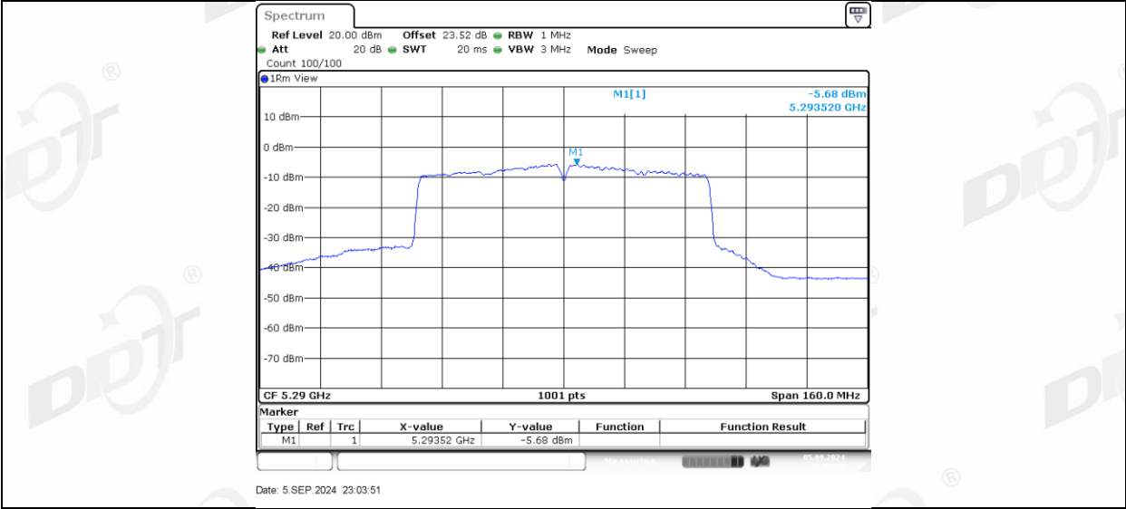
11AC80MIMO_Ant2_5290
