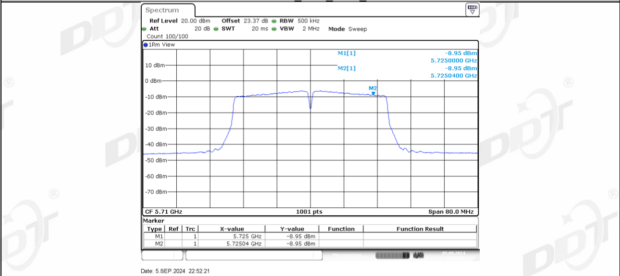
11AC40MIMO_Ant2_5710_UNII-3
