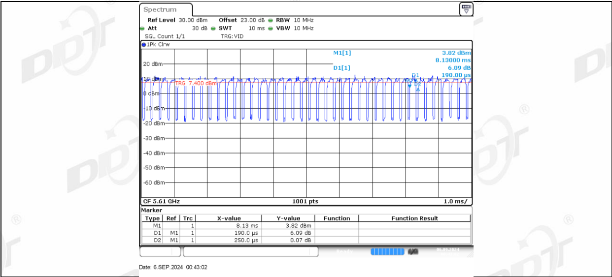
11AX80MIMO_Ant2_5610
