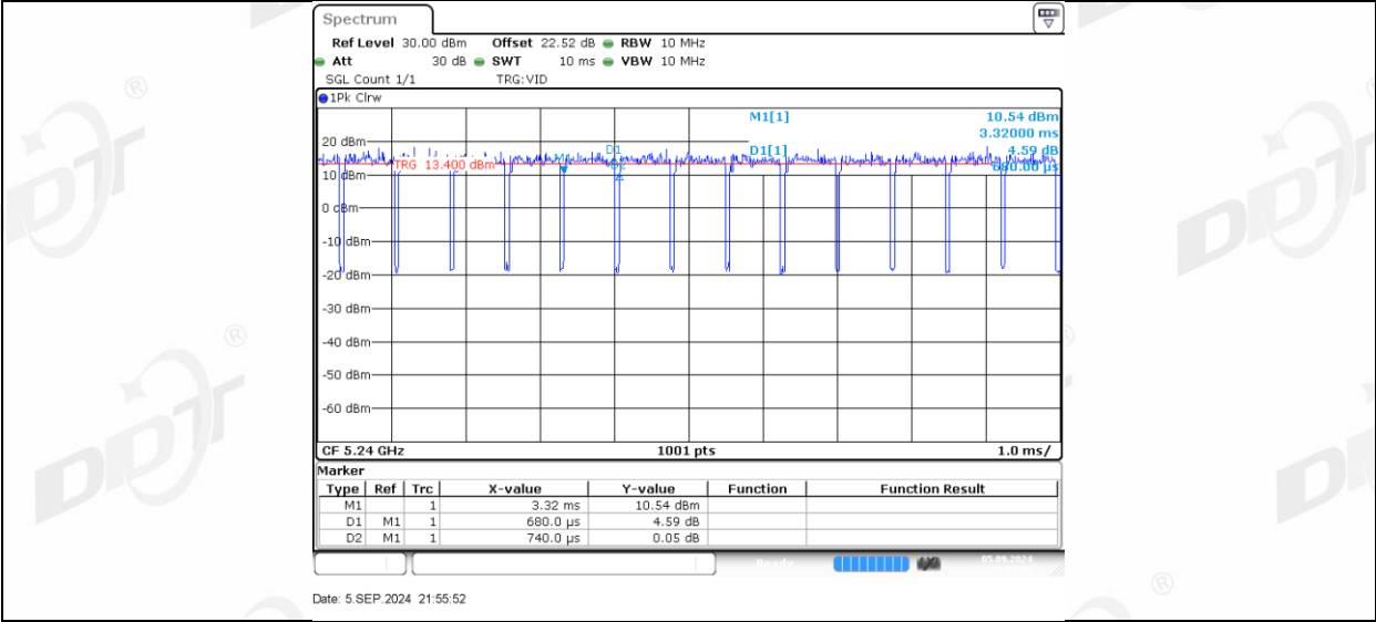
11AC20MIMO_Ant2_5240
