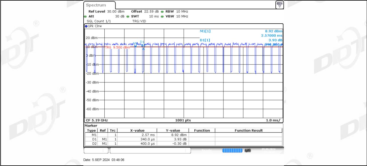
11N40MIMO_Ant2_5190
