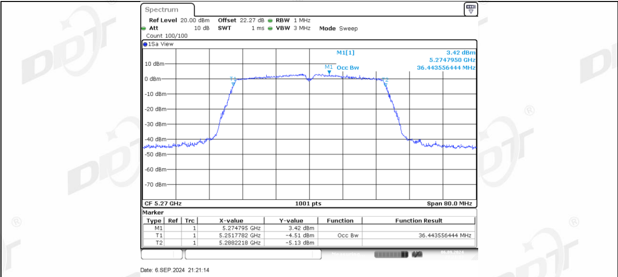
11AC40MIMO_Ant2_5270
