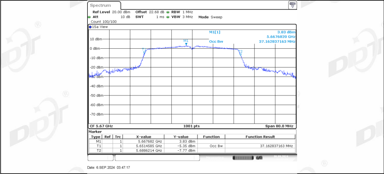
11N40MIMO_Ant2_5670
