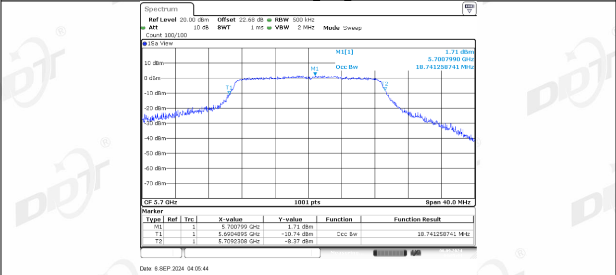
11AC20MIMO_Ant2_5700
